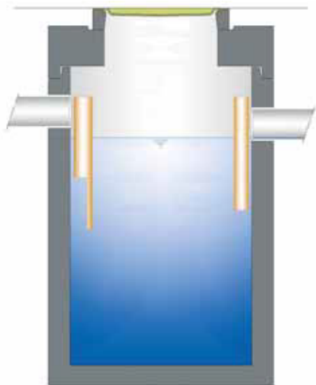
Vetafscheider met geïntegreerde slijpvang
