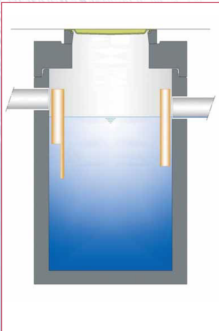
NEUTRA tip vetafscheider met geïntegreerde slibvang
