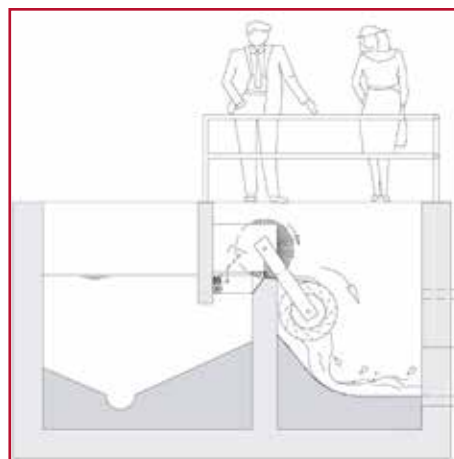
Een schematische doorsnede van de borstelinstallatie
